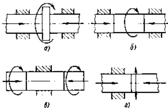
Рисунок 4 – Разновидности процесса сварки трением:
