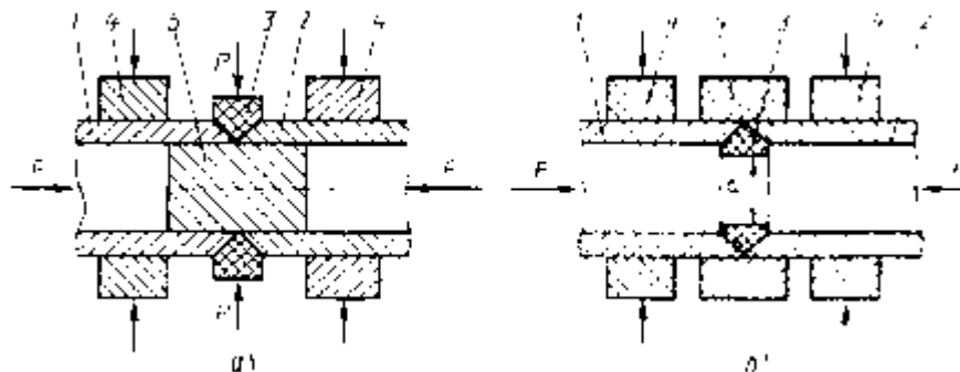
Рисунок 5 - Схема радиальной сварки трением:
