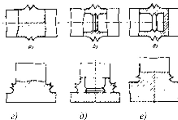
Рисунок 1 - Типы сварных соединений сварки трением:
