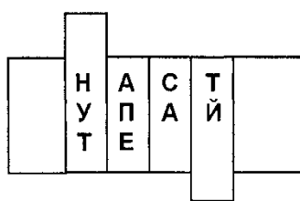
Рис. 1.2. Шифр "Скитала"
