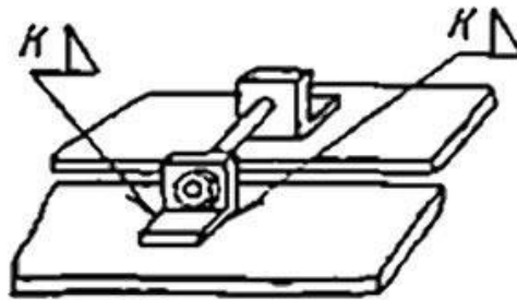
Приспособление для сварки: стяжка
