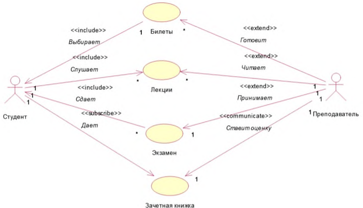
Рисунок 10. Модель студент сдает экзамен
