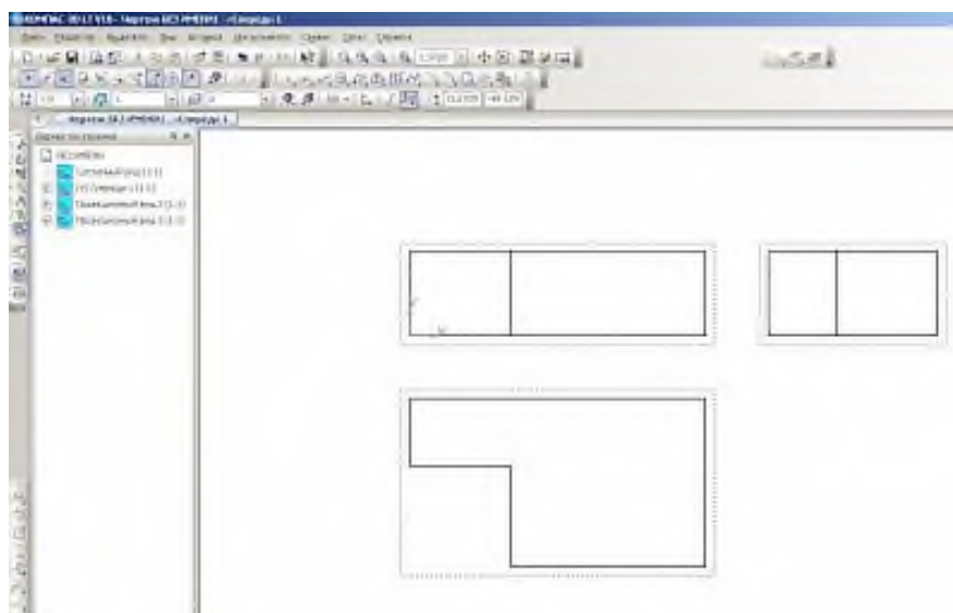
Рисунок 22 – Создание Объекта
