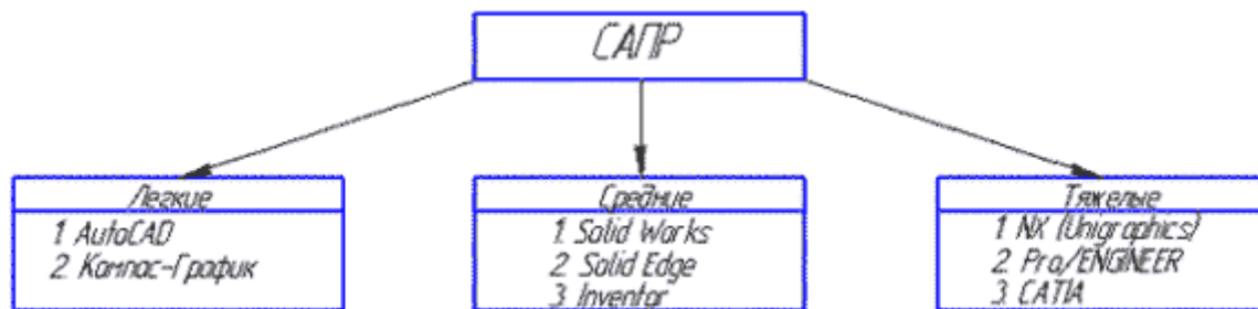
Рисунок 1 – Классификация САПР
