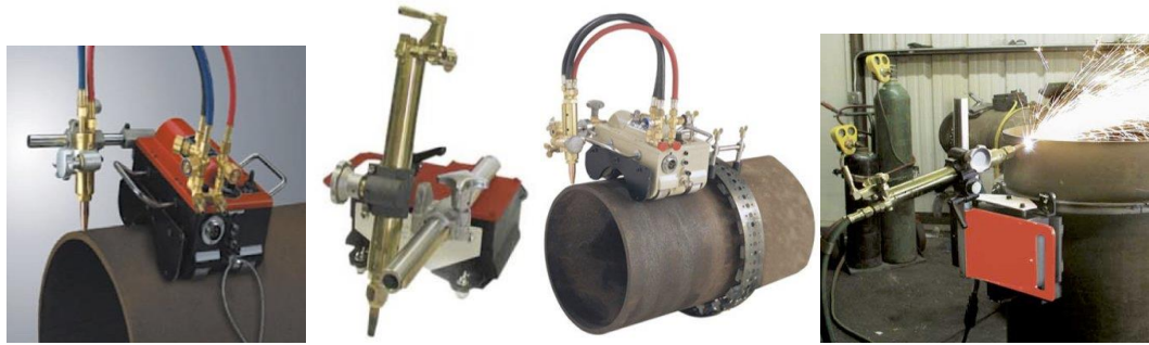
Рисунок 2. Машины для резки труб на магнитных колёсах: а – машина MagaPipe («GazCut», Китай); б – машина MiniMagXM («Mathey Dearman», США); в – позиционирование машин на магнитных колёсах на гибком кольцевом направляющем бандаже
