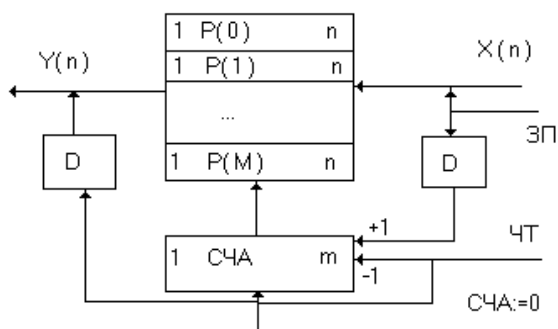
Рисунок 8.4 - Стековая память.
