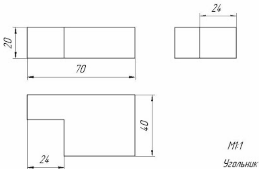
Рисунок 28 – Чертеж детали
